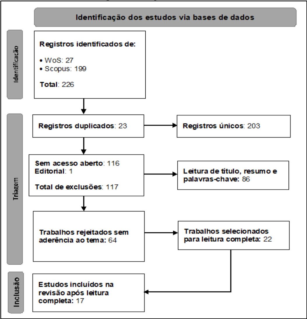
Figura 1: Diagrama Prisma
